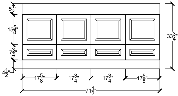
H-LINV 7222 BD-____-____-____ CENTER BOWL SINK
