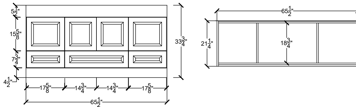
H-LINV 6622 BD-____-____-____ CENTER BOWL SINK
