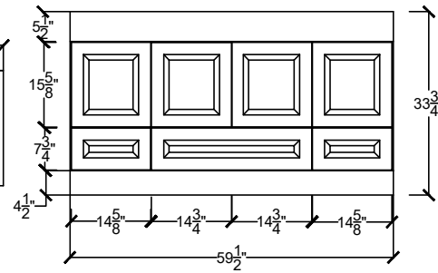
H-LINV 6022 BD-____-____-____ CENTER BOWL SINK
