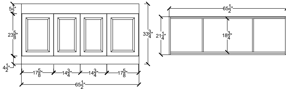
H-LINV 6622-____-____-____ CENTER BOWL SINK
