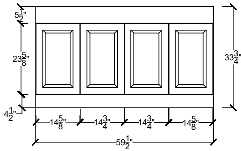
H-LINV 6022-____-____-____ CENTER BOWL SINK
