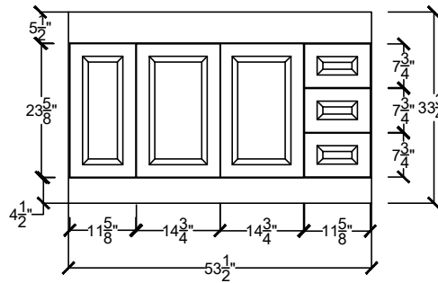
H-LINV 5422 3DL-____-____-____ OR H-LINV 5422 3DR-____-____-____
