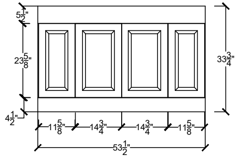
H-LINV 5422-____-____-____ CENTER BOWL SINK
