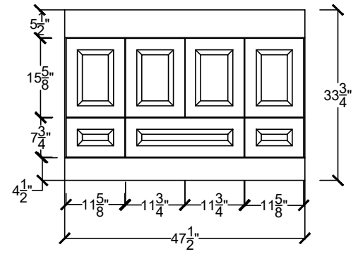
H-LINV 4822 BD-____-____-____ CENTER BOWL SINK
