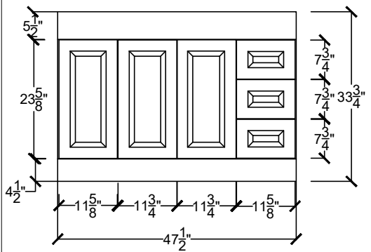
H-LINV 4822 3DL-____-____-____ OR H-LINV 4822 3DR-____-____-____
