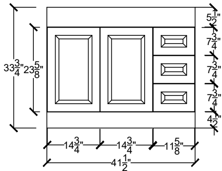
H-LINV 4222 3DL-_____-_____-_____ OR H-LINV 4222 3DR-_____-_____-_____
