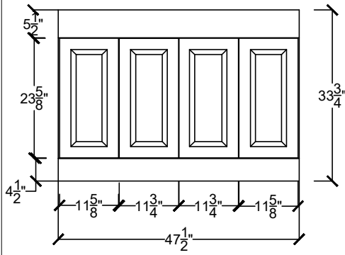
H-LINV 4822-____-____-____ CENTER BOWL SINK
