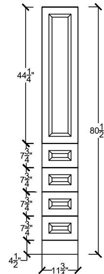
H-LINTC 1222-4D-
