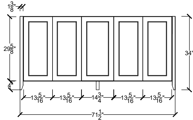
DIAV 7222-____-____-____ DOUBLE BOWL SINK
