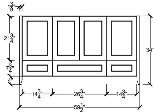
DIAV 6022 BD-____-____-____ CENTER BOWL SINK
