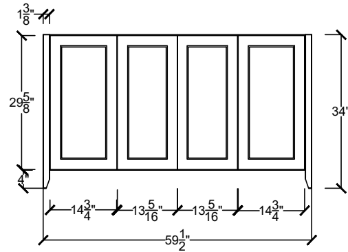
DIAV 6022-____-____-____ CENTER BOWL SINK
