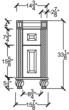
ANAS 1522-1D- - - - -
