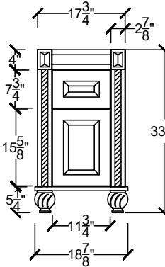
ANAS 1822-1D- - - - -
