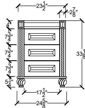
ANAS 2422-3D- - - - -
