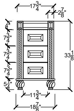
ANAS 1822-3D- - - - -
