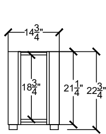
ANAS 1522-1D- - - - -
